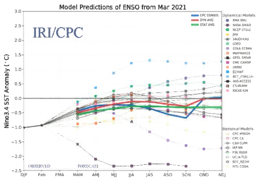
Figura 13 Pronóstico de las anomalías en la temperatura en la superficie del océano para la región de El Niño
