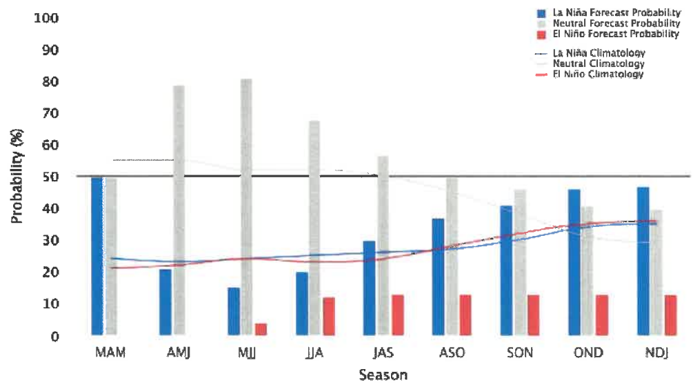
Figura 14 Probabilidad de condiciones de El niño y La niña
